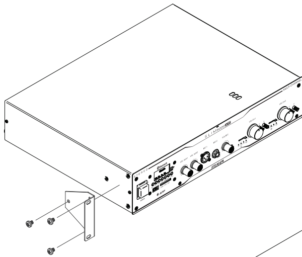
FIXADORES LATERAIS
