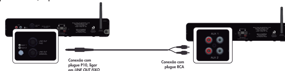
Exemplo de ligação ideal de um Slim em outro amplificador / Slim.
