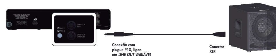
Exemplo de ligação ideal de um Slim em um subwoofer.
